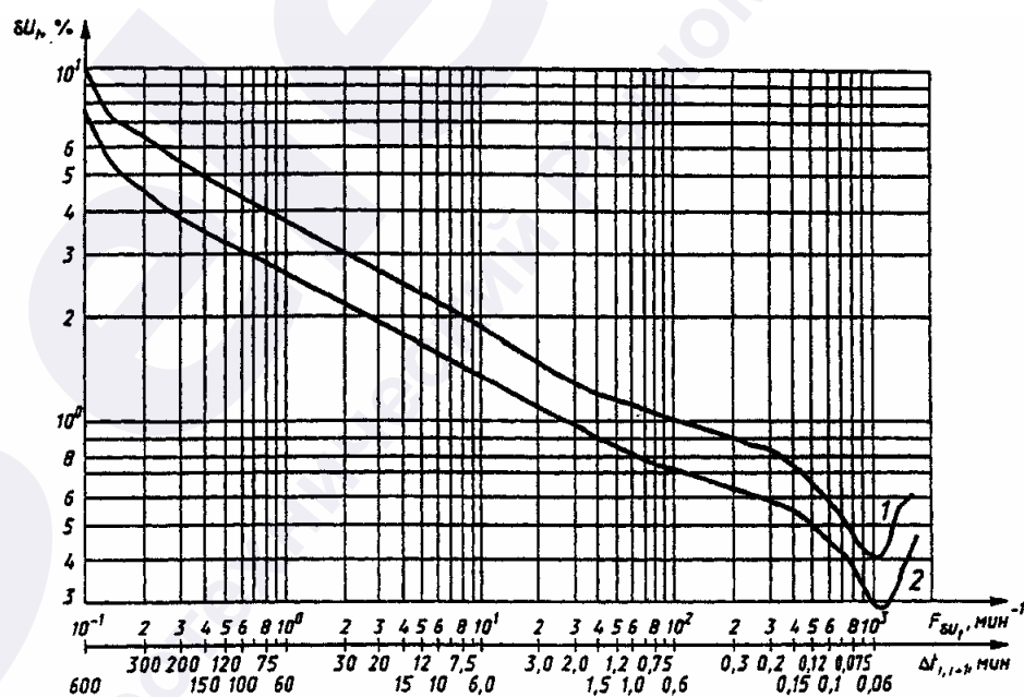
Рисунок 1. Предельно допустимые размахи изменения напряжения в зависимости от частоты повторения изменений напряжения за минуту для колебаний напряжения, имеющих форму меандра
